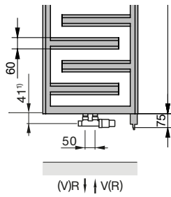
Elektrická prevádzka: s vstavanou el. vykurov. tyčou IHD
