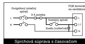
Schéma zapojenia
