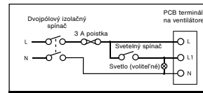
Sprchová súprava s časovačom
