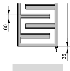
Elektrická prevádzka: s vstavanou el. vykurov. tyčou IHE
