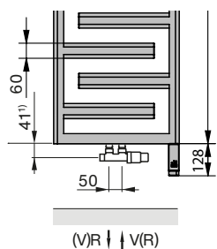
Elektrická prevádzka: s vstavanou el. vykurov. tyčou IHC
