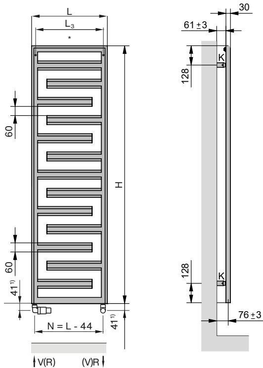
Kombinovaná prevádzka: s vstavanou el. vykurov. tyčou IHD
