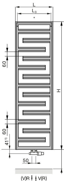
Kombinovaná prevádzka: s vstavanou el. vykurov. tyčou IHC
