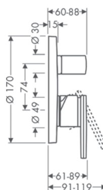
Páková ruční vanová baterie s podomítkovou instalací, s pákovou rukojetí a se zabudovanou ochranou proti zpětnému toku
