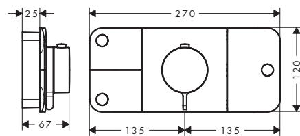
Modul termostatu Axor One s podomítkovou instalací, pro 3 spotřebiče
