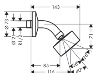
Horní sprcha 75 1jet EcoSmart se sprchovým ramenem
